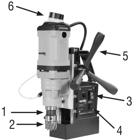
Fig. 1 – Componentes
